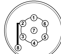
Johtojen liittyminen 7-napaiseen pistorasiaan
